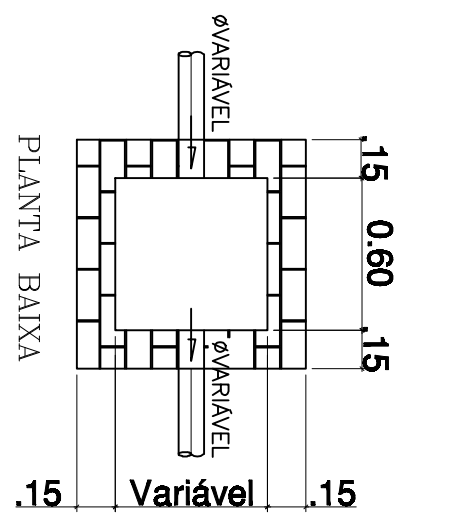
DET. CAIXA DE AGUAS PLUVIAS ESCALA 1/25
