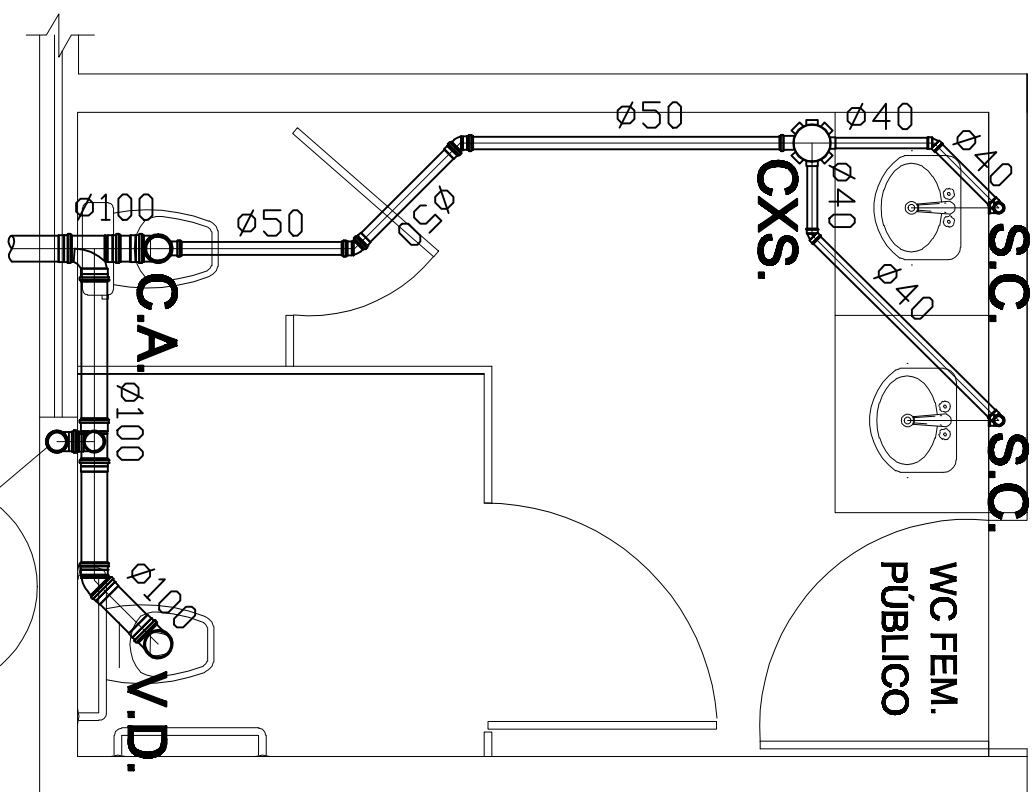
DETALHE 8=9 ESC. 1/25
