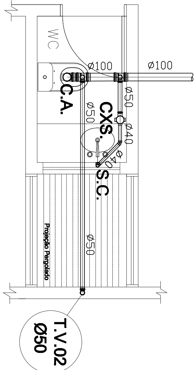
DETALHE 2 ESC. 1/25
