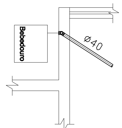
DETALHE 11 ESC. 1/25
