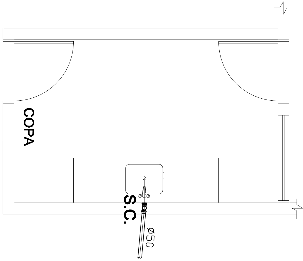
DETALHE 5 ESC. 1/25
