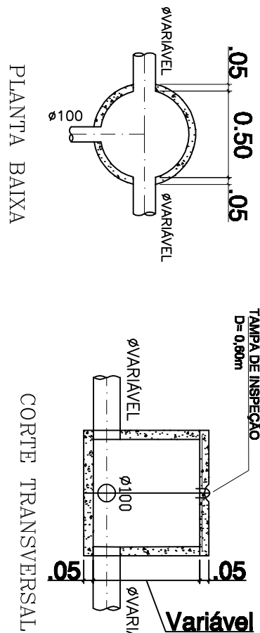
DET. CAIXA DE INSPEÇÃO - PRÉ-MOLDADA ESCALA 1/25
